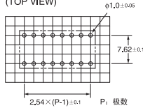
印刷基板加工尺寸 (TOP VIEW)
