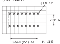
印刷基板加工尺寸 (TOP VIEW)
